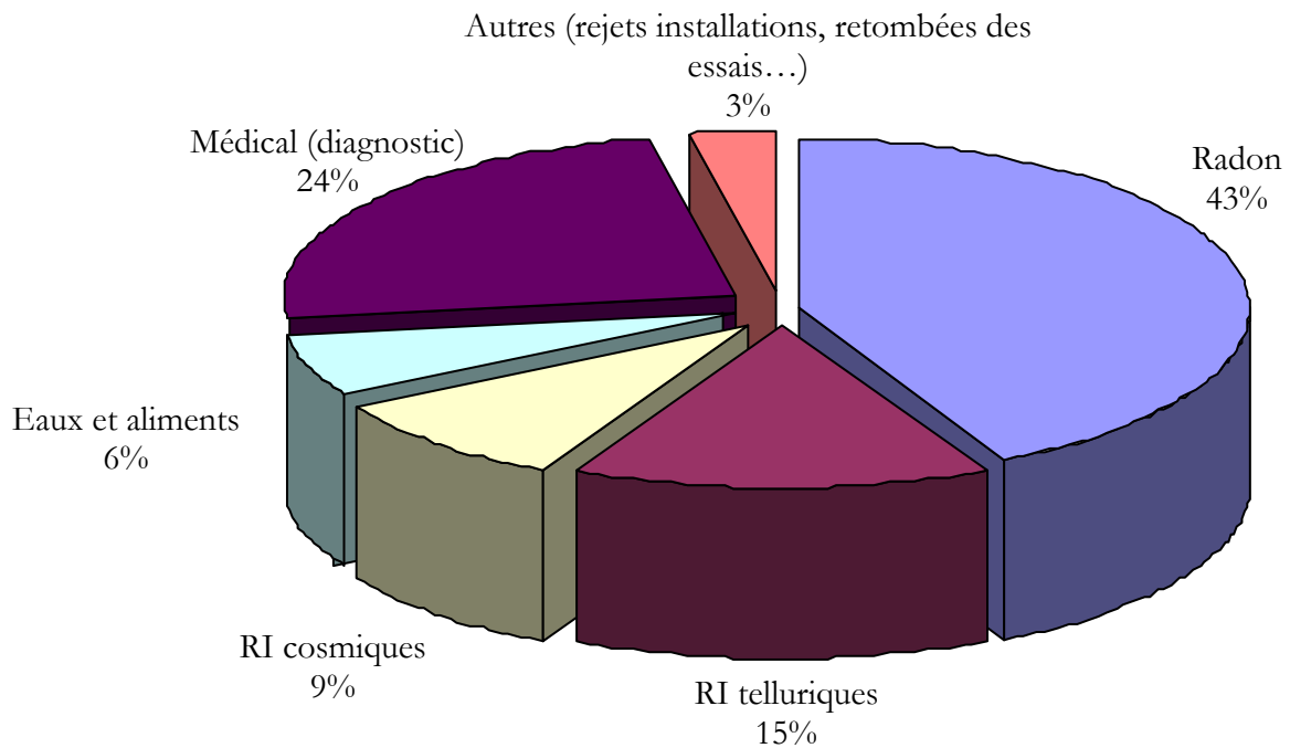
Exposition aux rayonnements ionisants de la population en France (source IRSN, estimation en 2005) Doses annuelles totales = 3,3 mSv/an par personnes en moyenne
